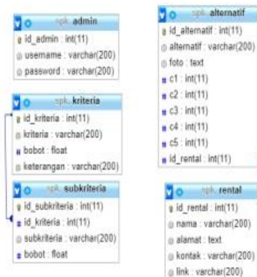
Gambar.6 Relasi database
